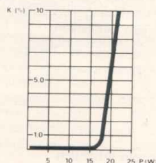
Abb. 2 zeigt den typischen Verlauf der Klirrfaktor-kurve des Boosters PA 80. Die Nennleistung von 4x15 Watt Sinus n. DIN 45500 (4x20 Watt n. DIN 45324) und der äußerst geringe Klirrfaktor sind ein Maßstab für Leistung und Qualität.
